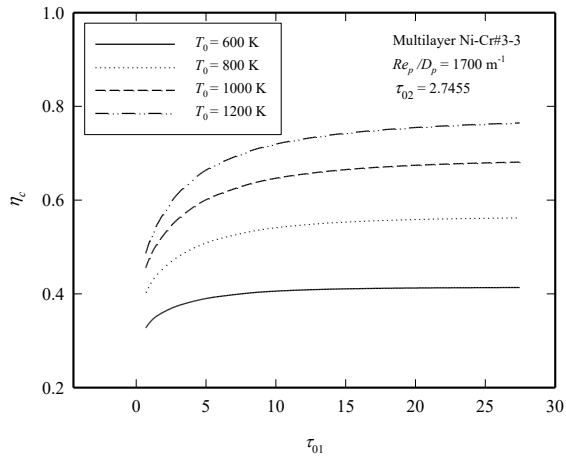
รูปที่ 1 ความสัมพันธ์ของประสิทธิภาพการแปลงรังสี ความร้อนกับความหนาเชิงแสงของชั้นวัสดุพลาสมา
